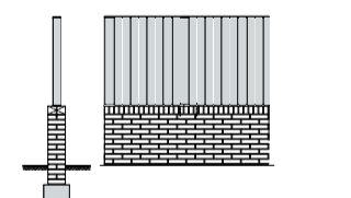
#2 Lage tuinmuur met aluminium ca. 1800 hoog Schaal 1:100
