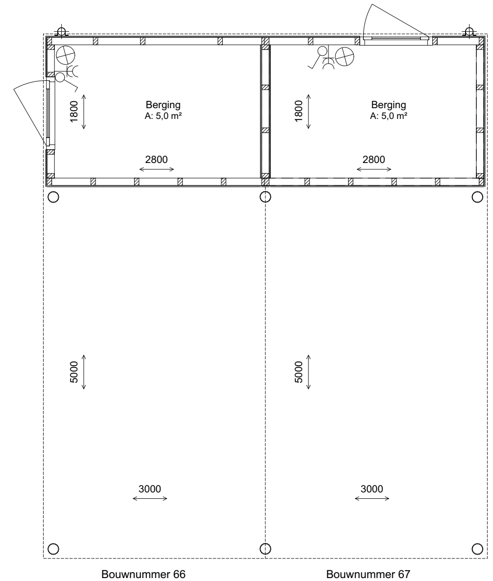
plattegrond 1:50
