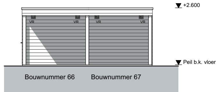
voorgevel 1:100
