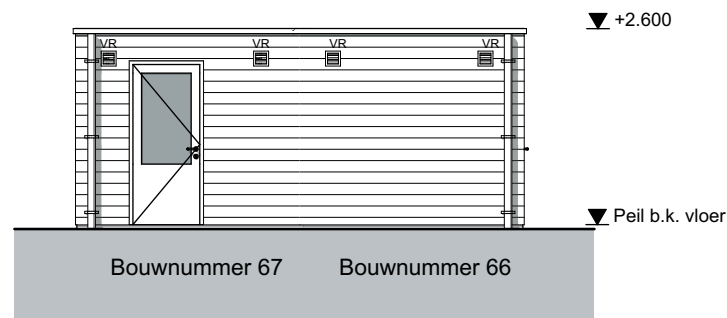
achtergevel 1:100
