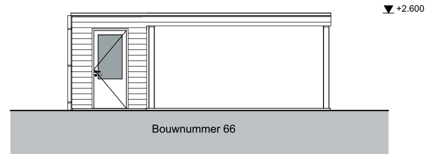
linkergevel 1:100
