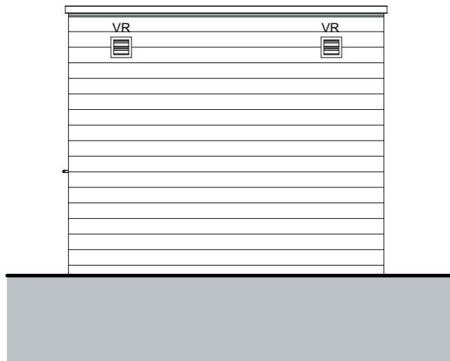
rechtergevel 1:50
