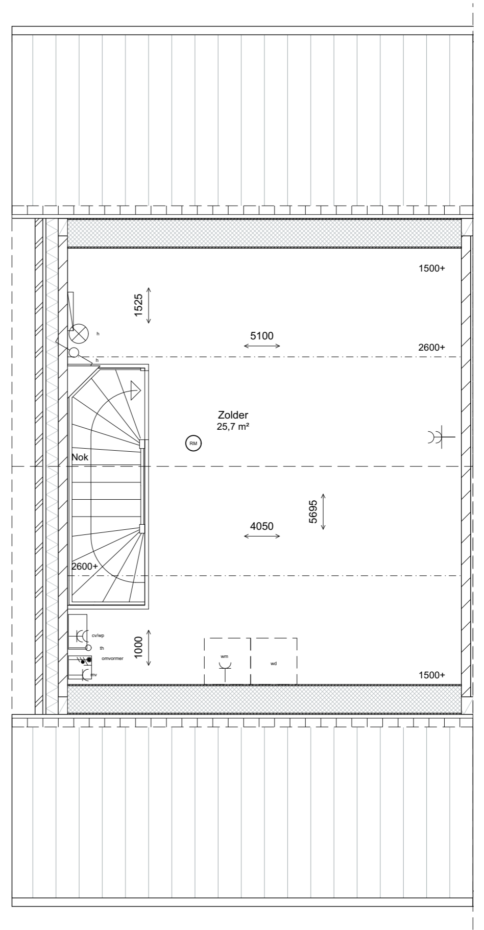
tweede verdieping 1:50
