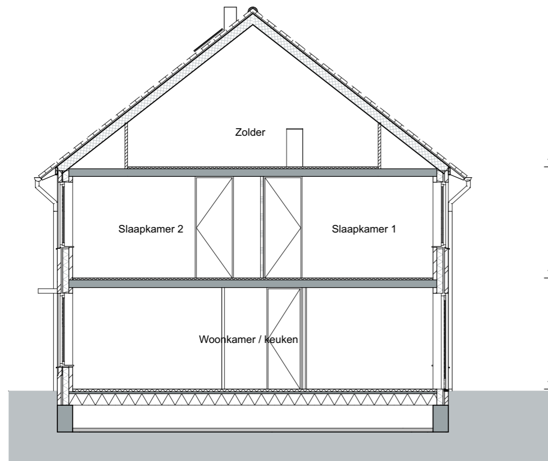
doorsnede A-A 1:100
