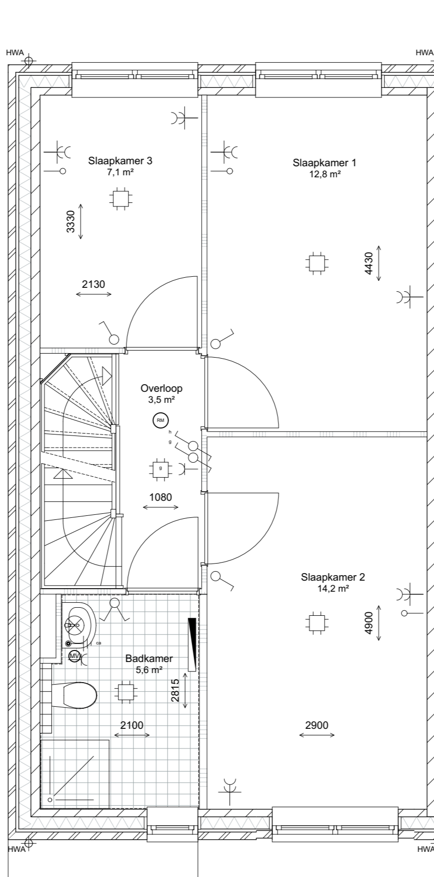
eerste verdieping 1:50
