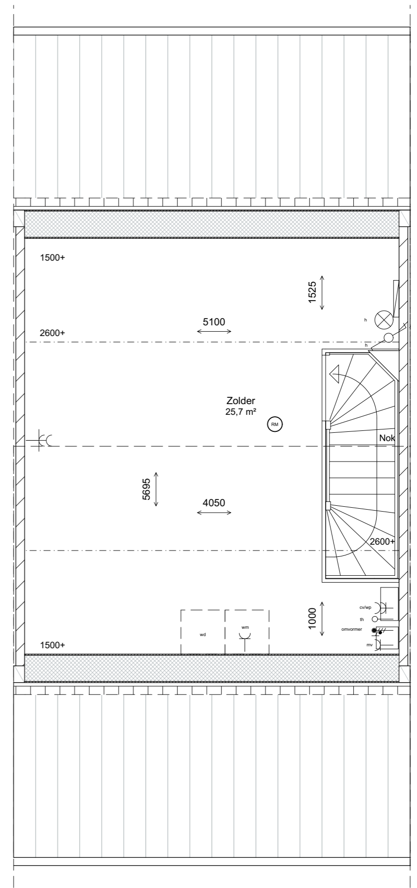
tweede verdieping 1:50
