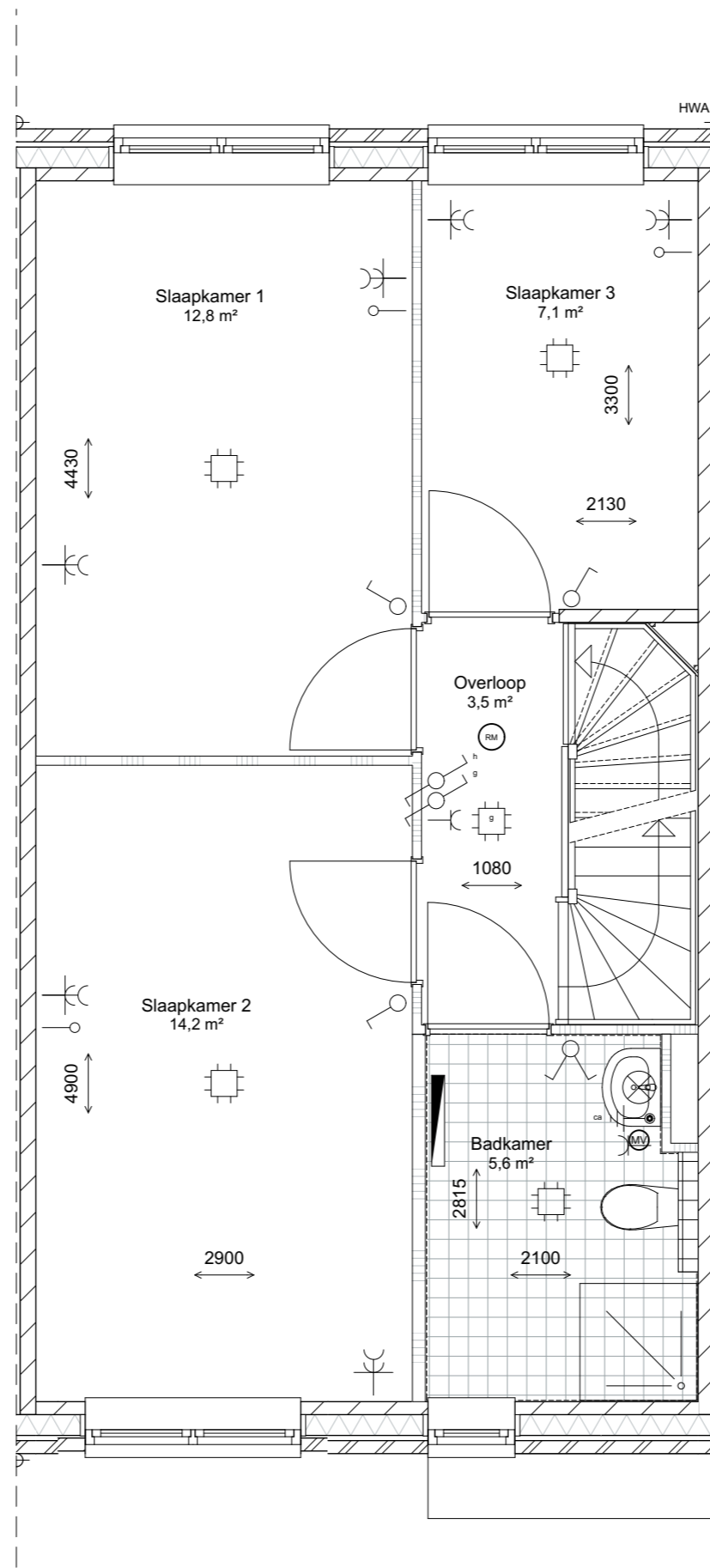
eerste verdieping 1:50
