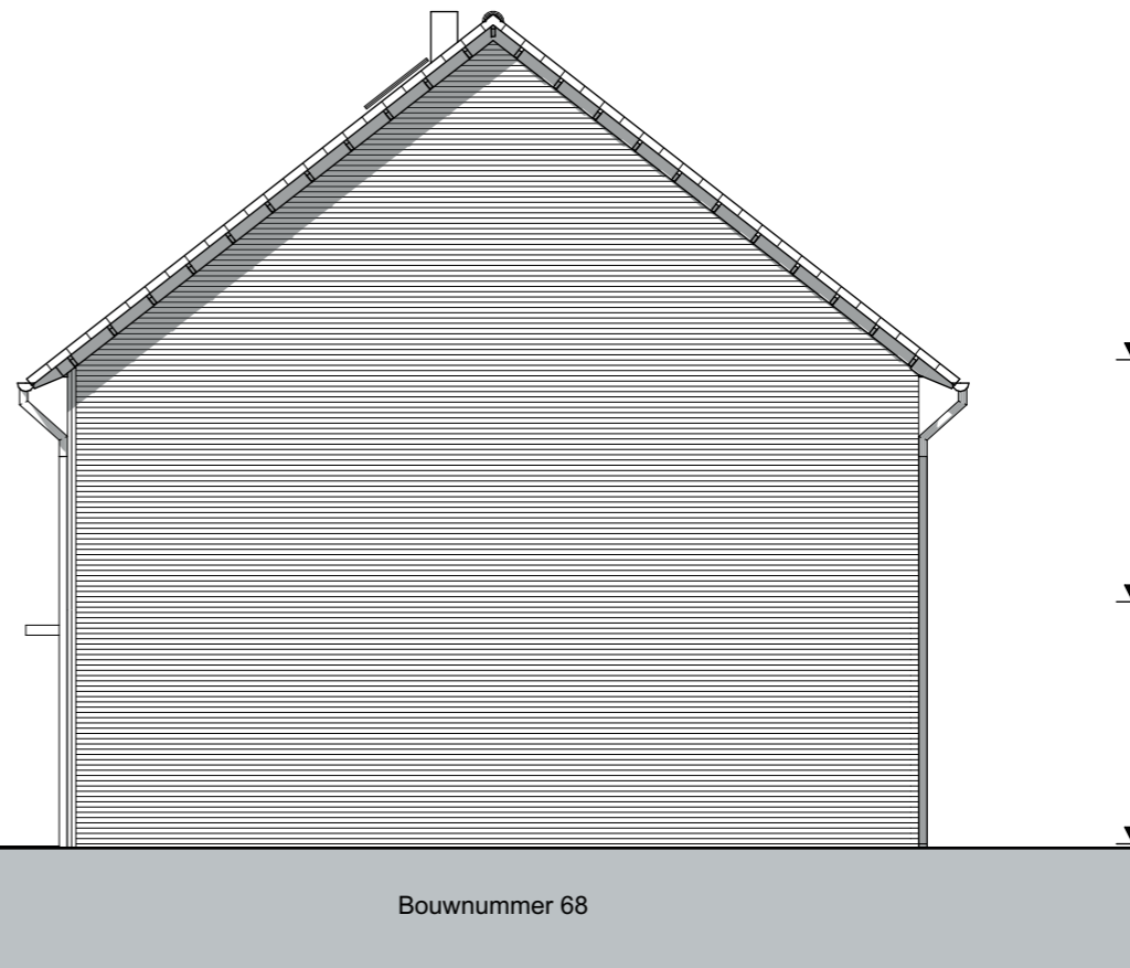
Rechter zijgevel 1:100
