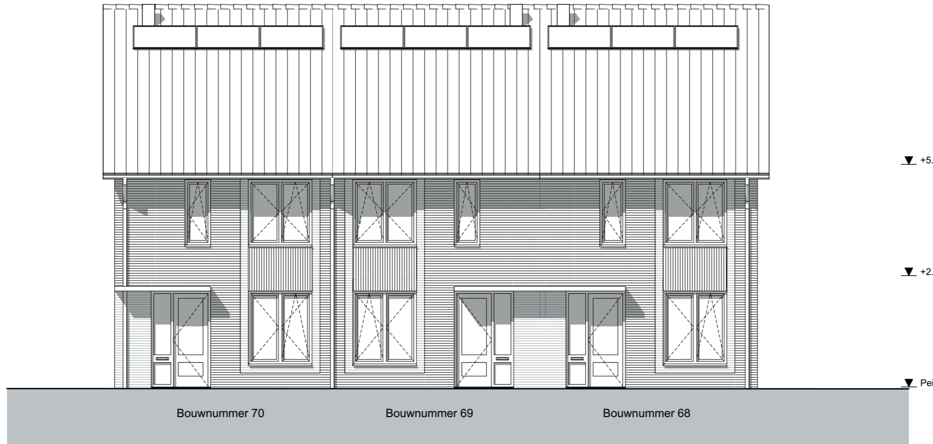
voorgevel 1:100
