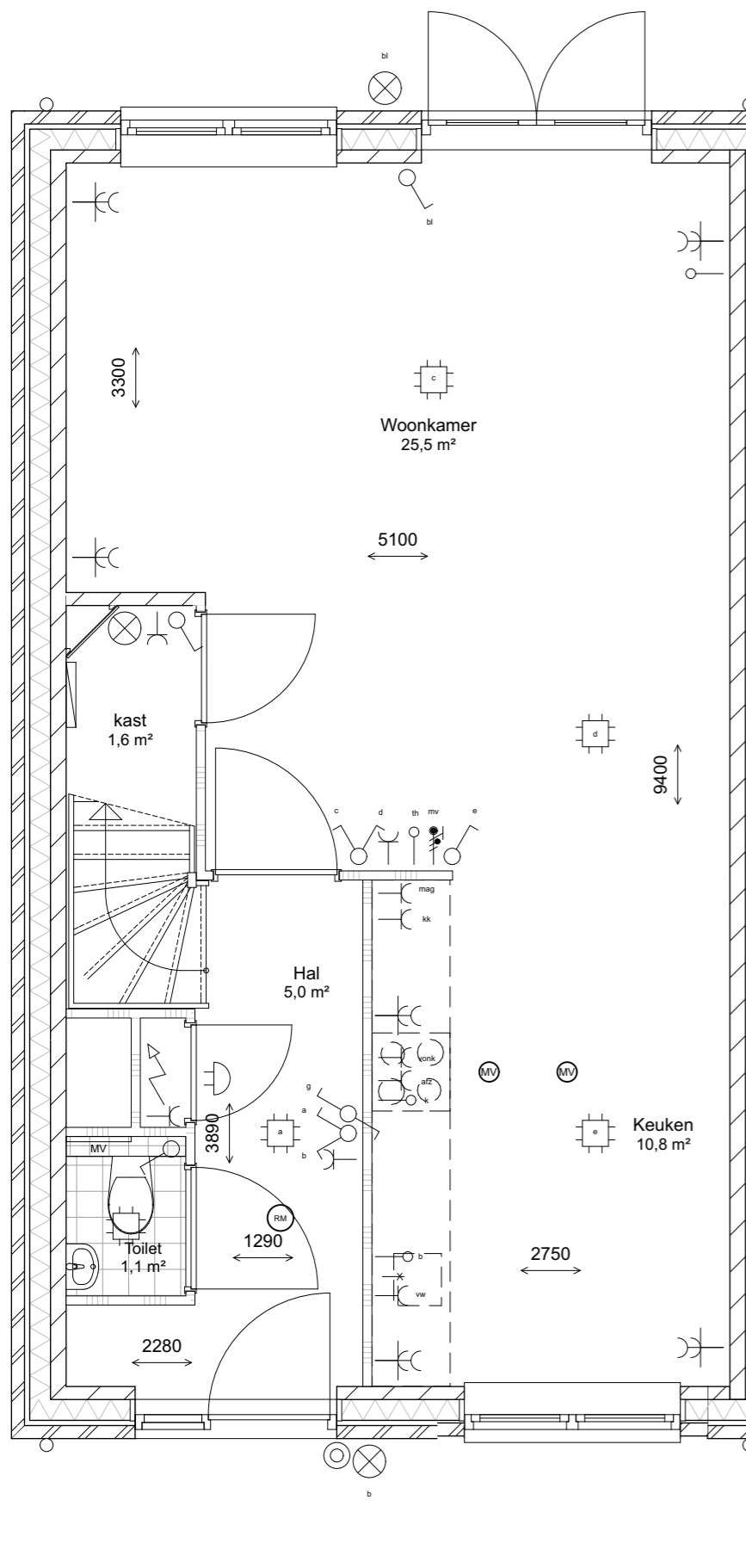
begane grond 1:50
