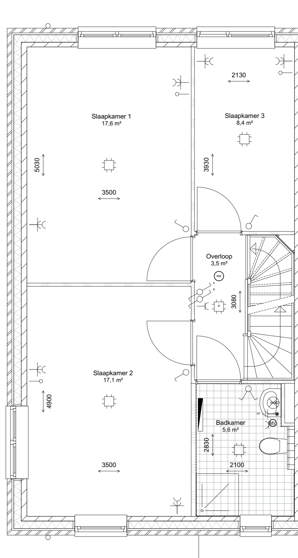
eerste verdieping 1:50
