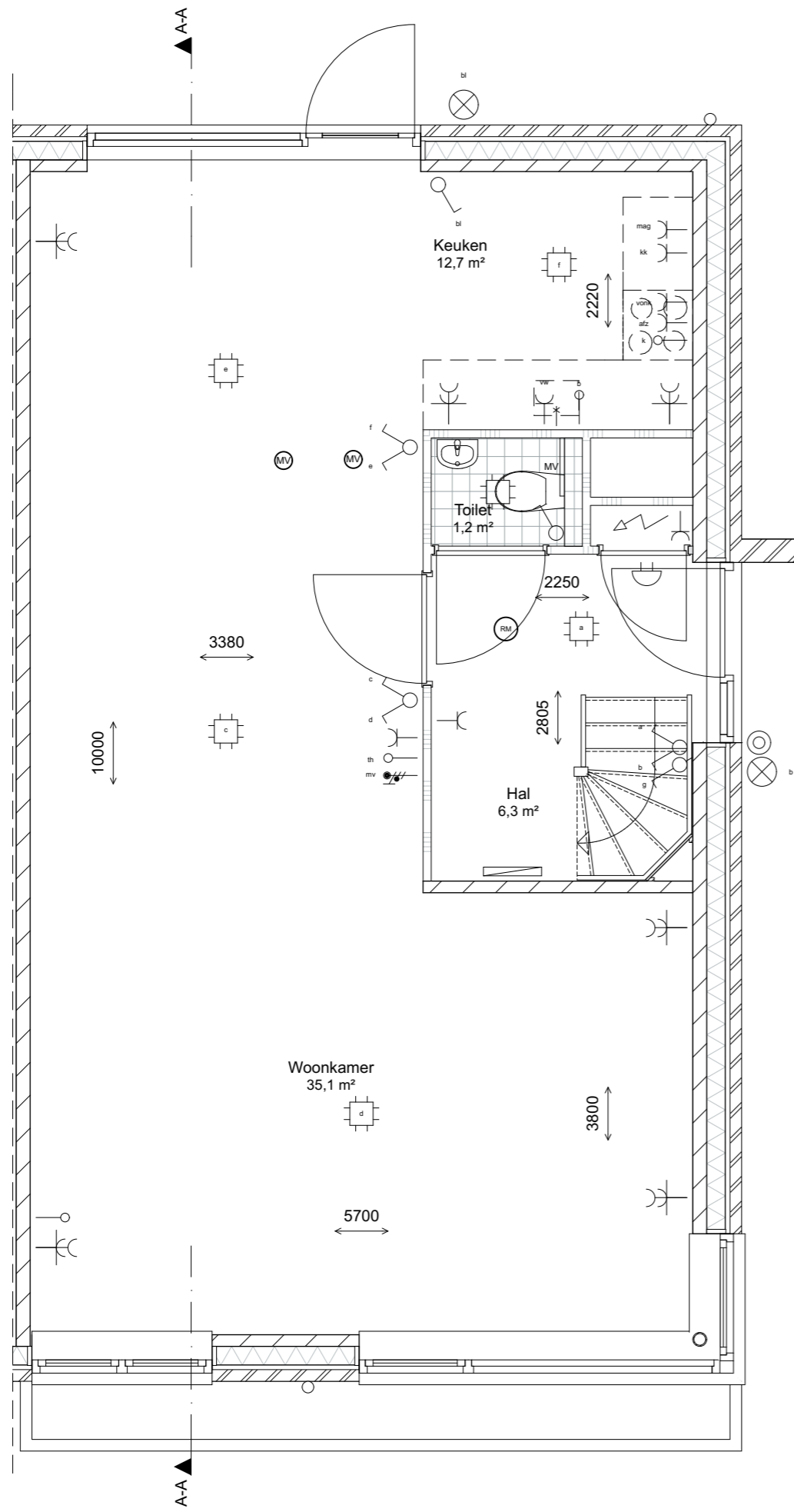
begane grond 1:50
