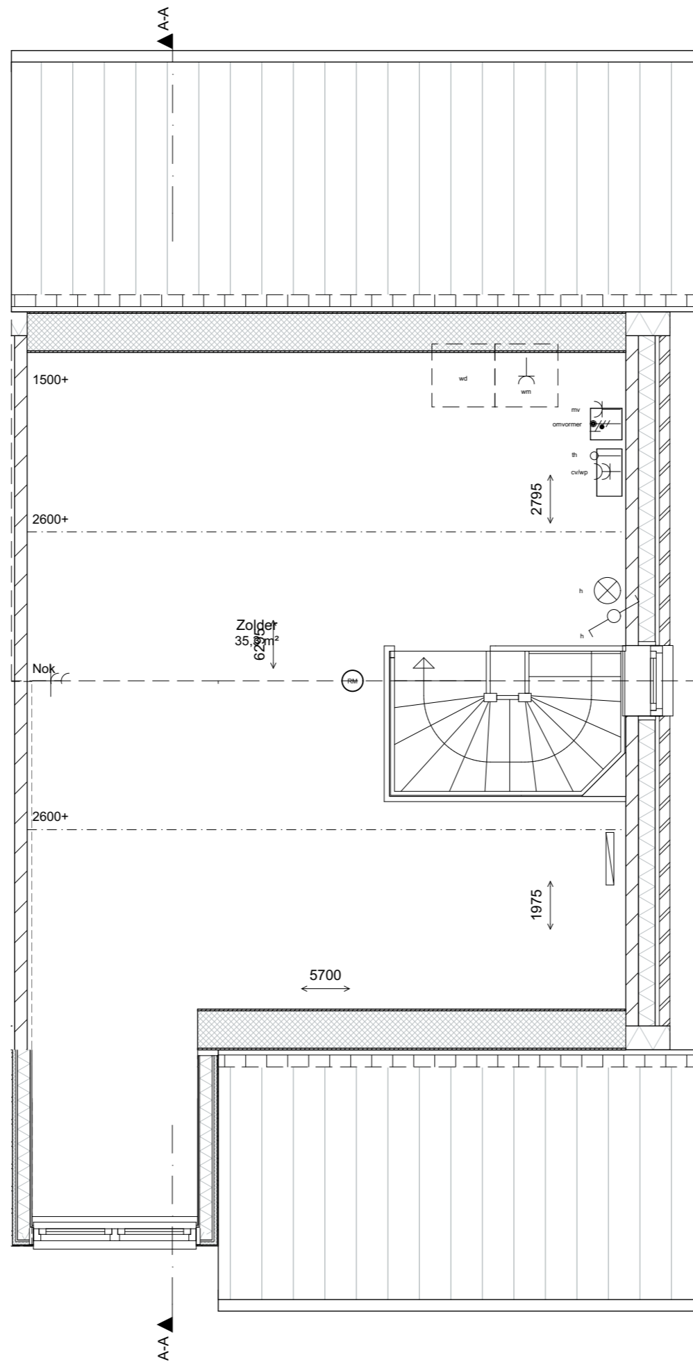
tweede verdieping 1:50
