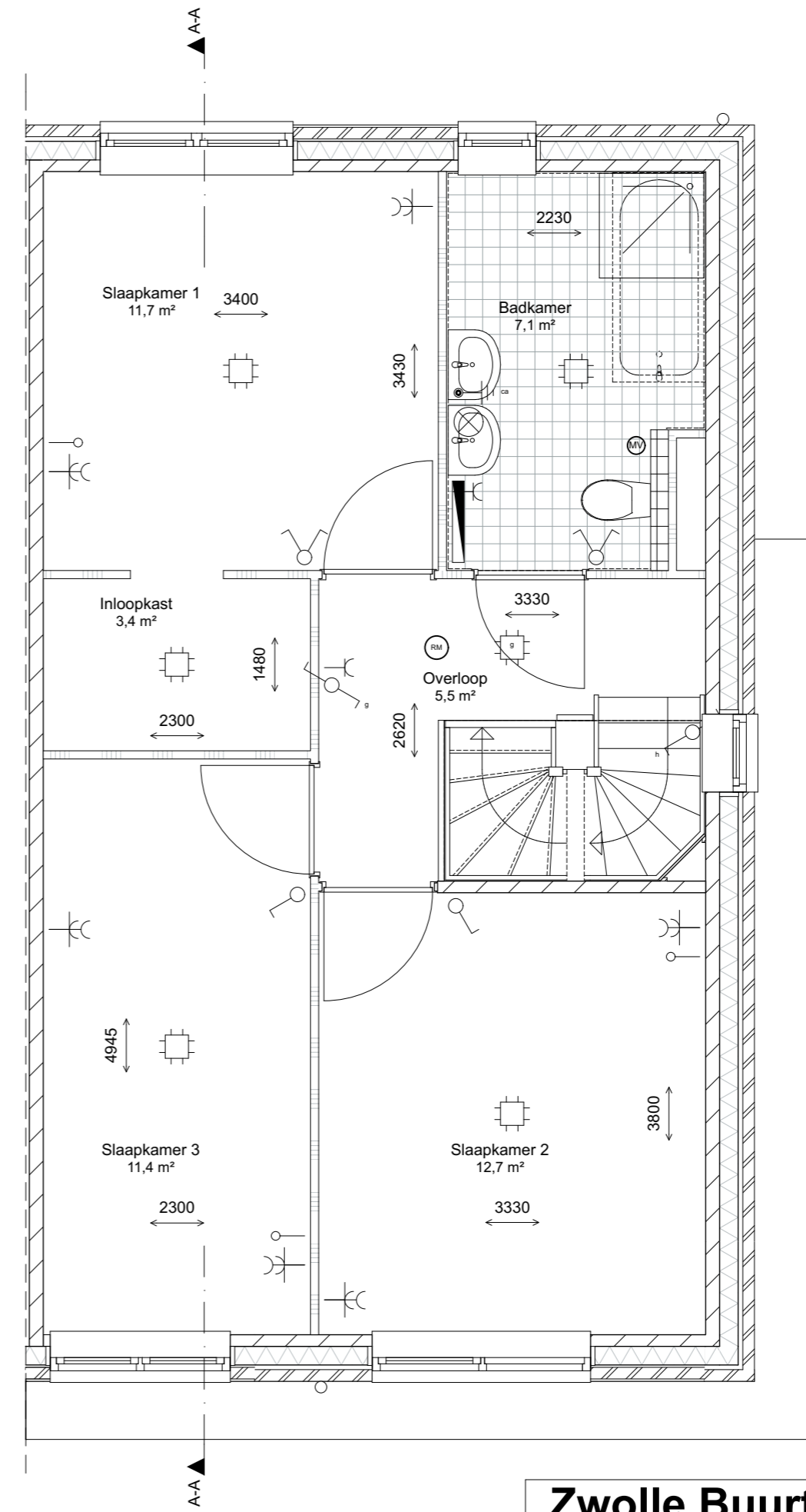
eerste verdieping 1:50
