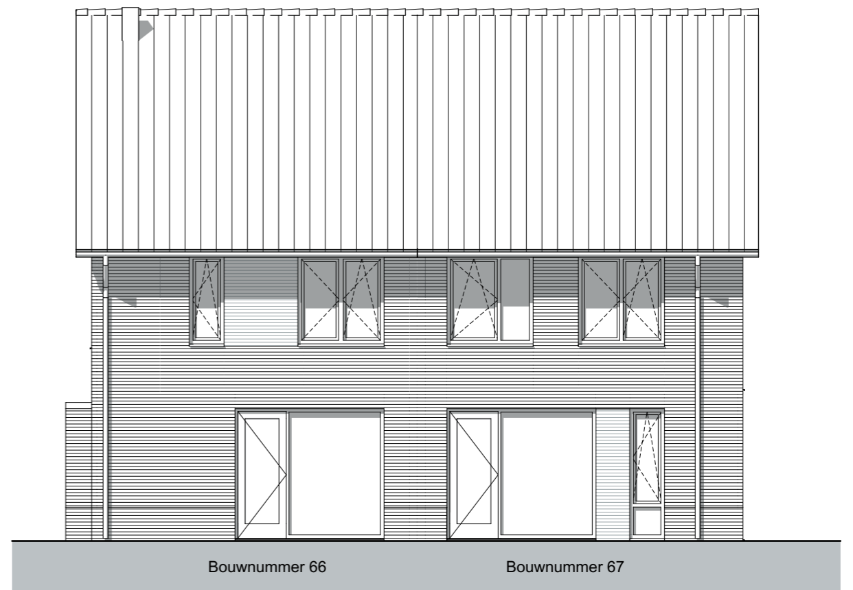
achtergevel 1:100
