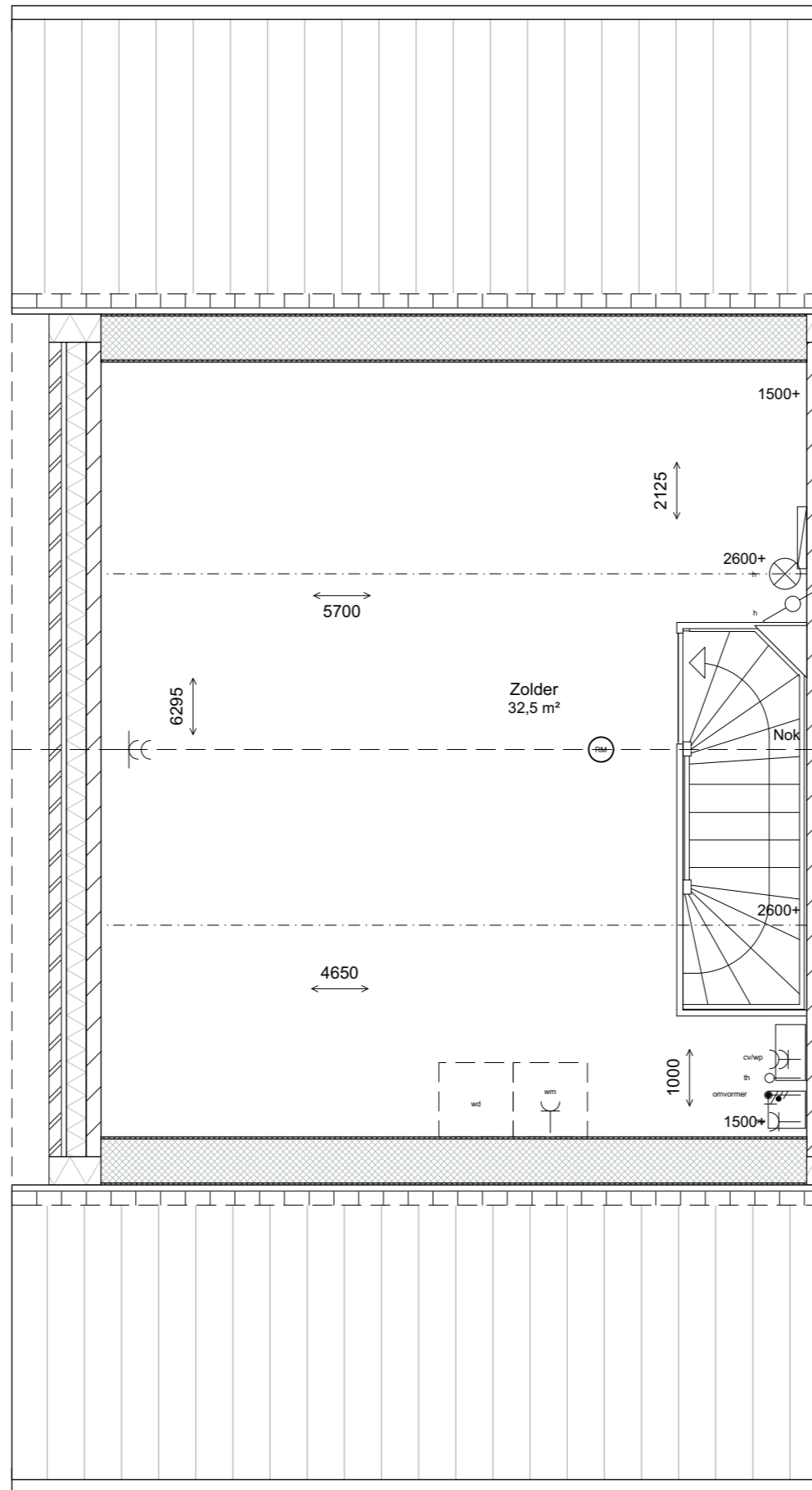
tweede verdieping 1:50
