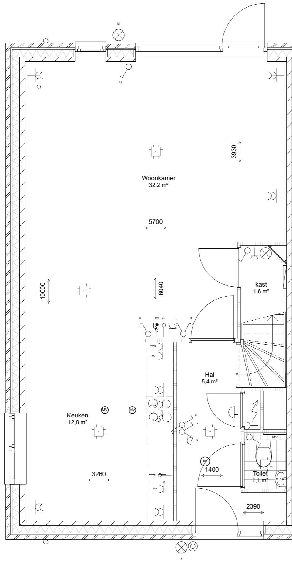
begane grond 1:50
