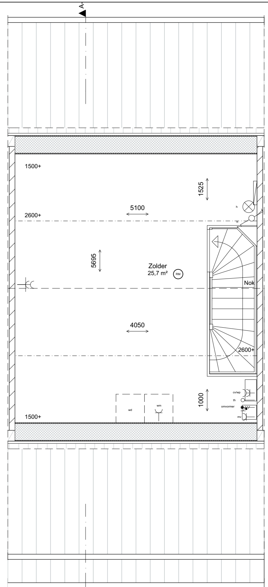
tweede verdieping 1:50
