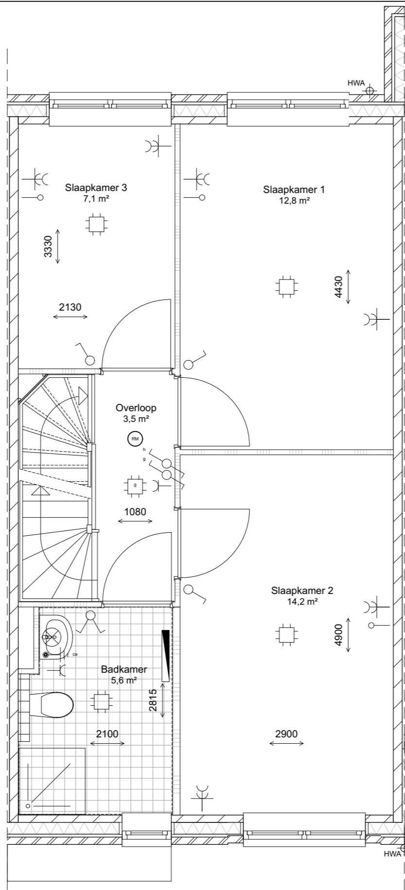
eerste verdieping 1:50
