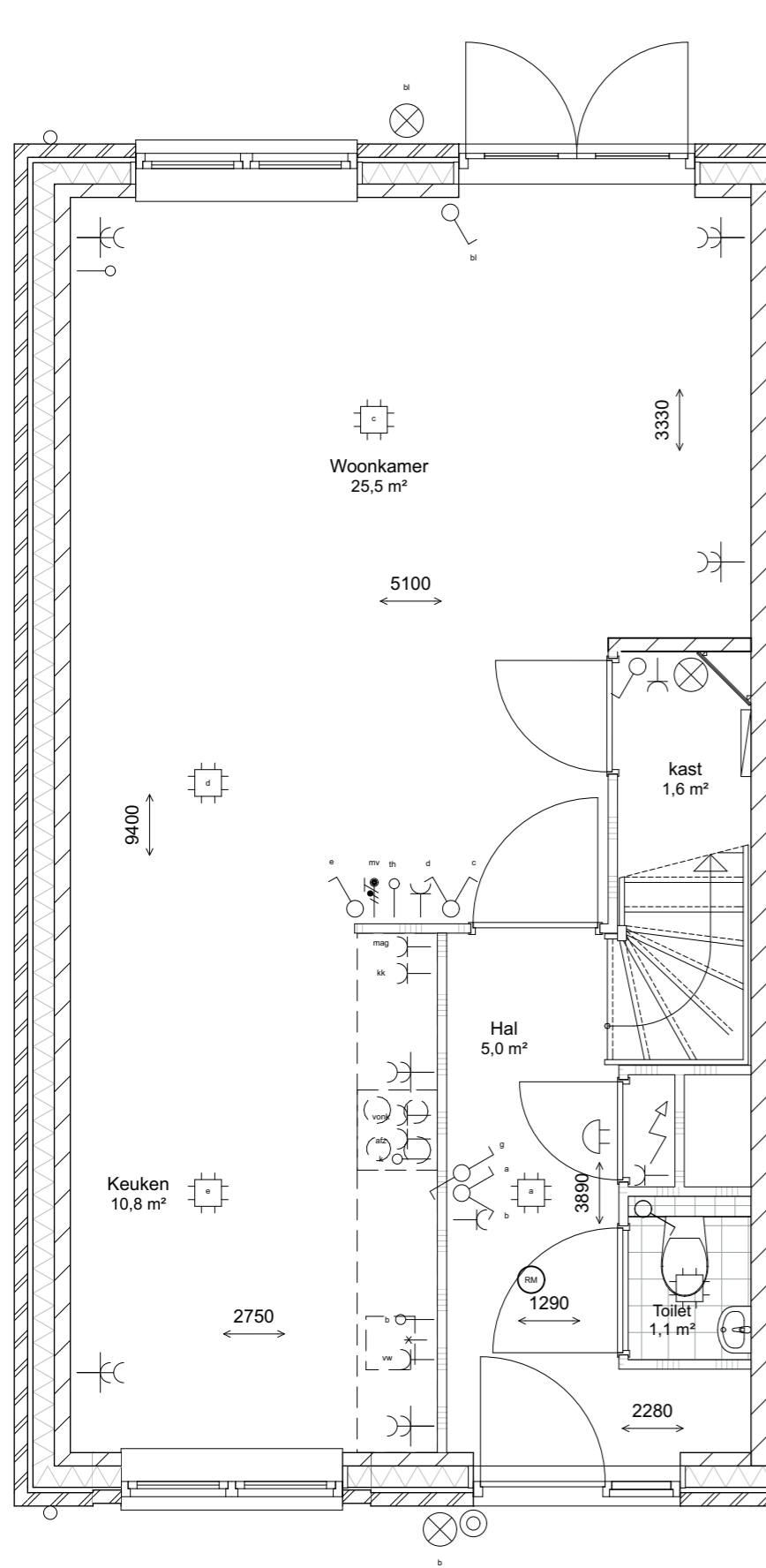
begane grond 1:50
