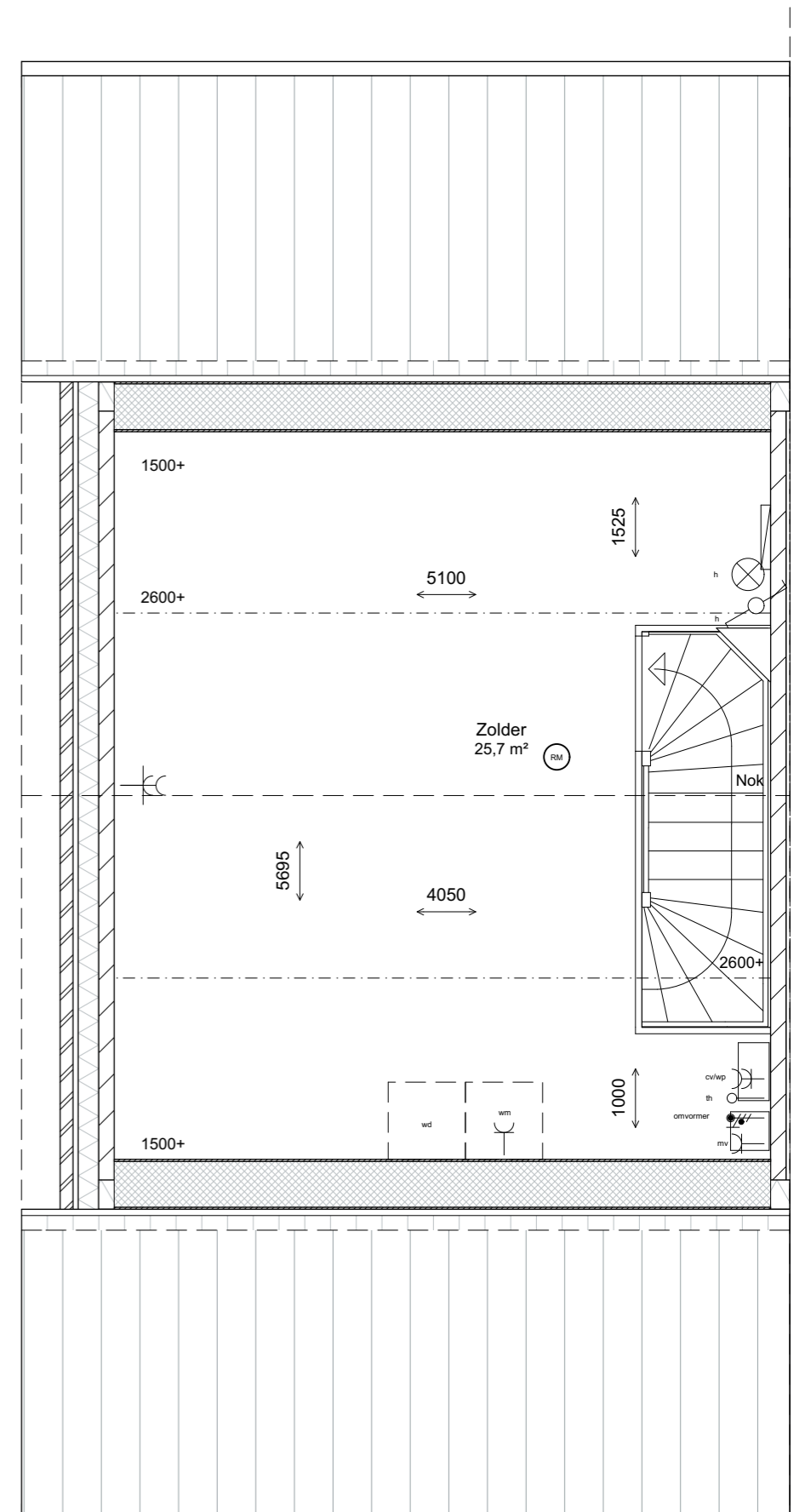
tweede verdieping 1:50
