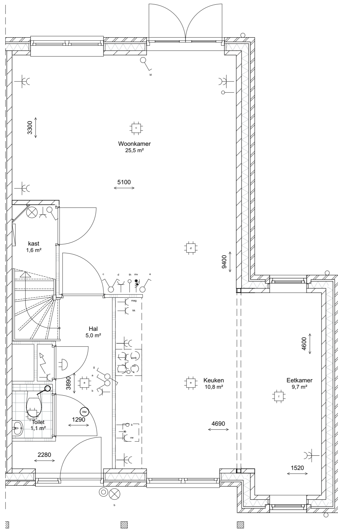
begane grond 1:50
