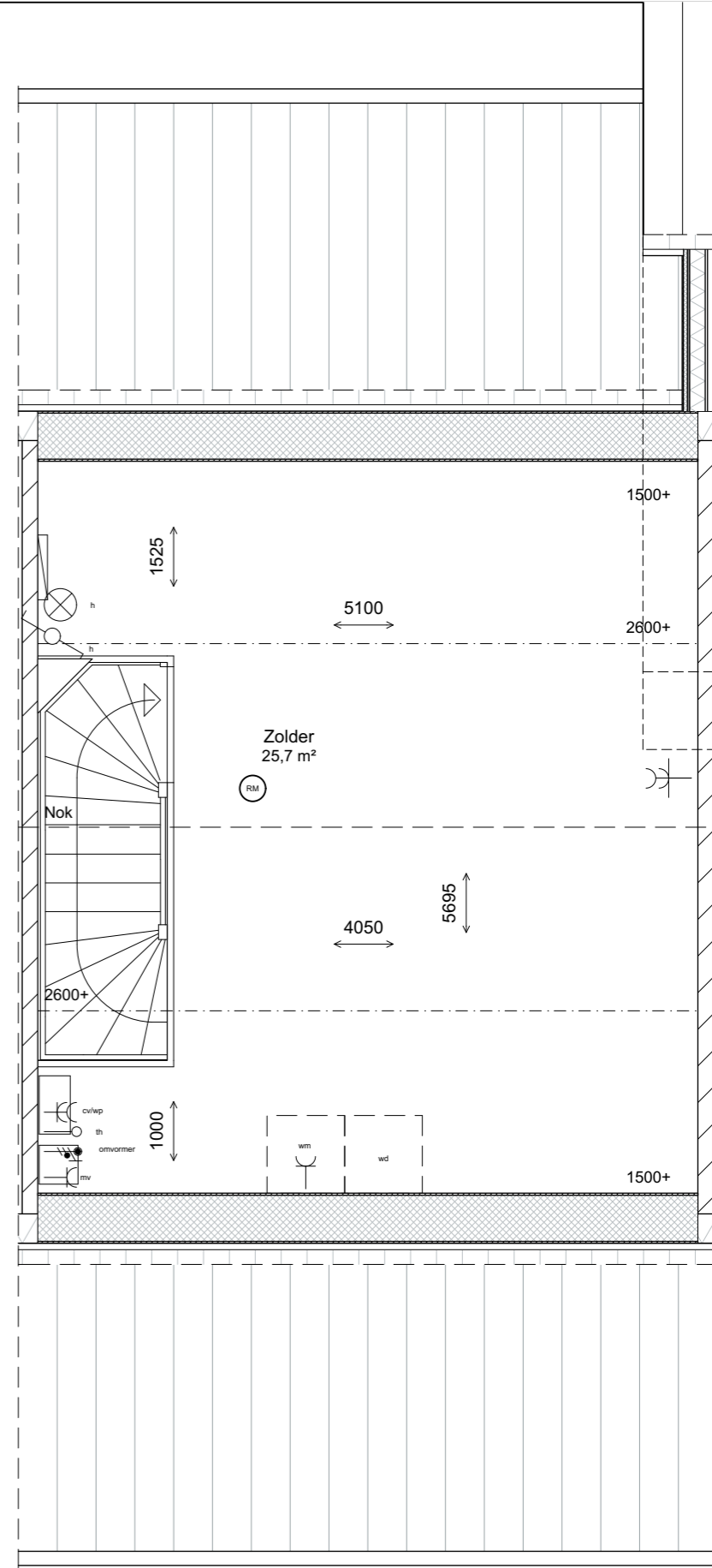
tweede verdieping 1:50
