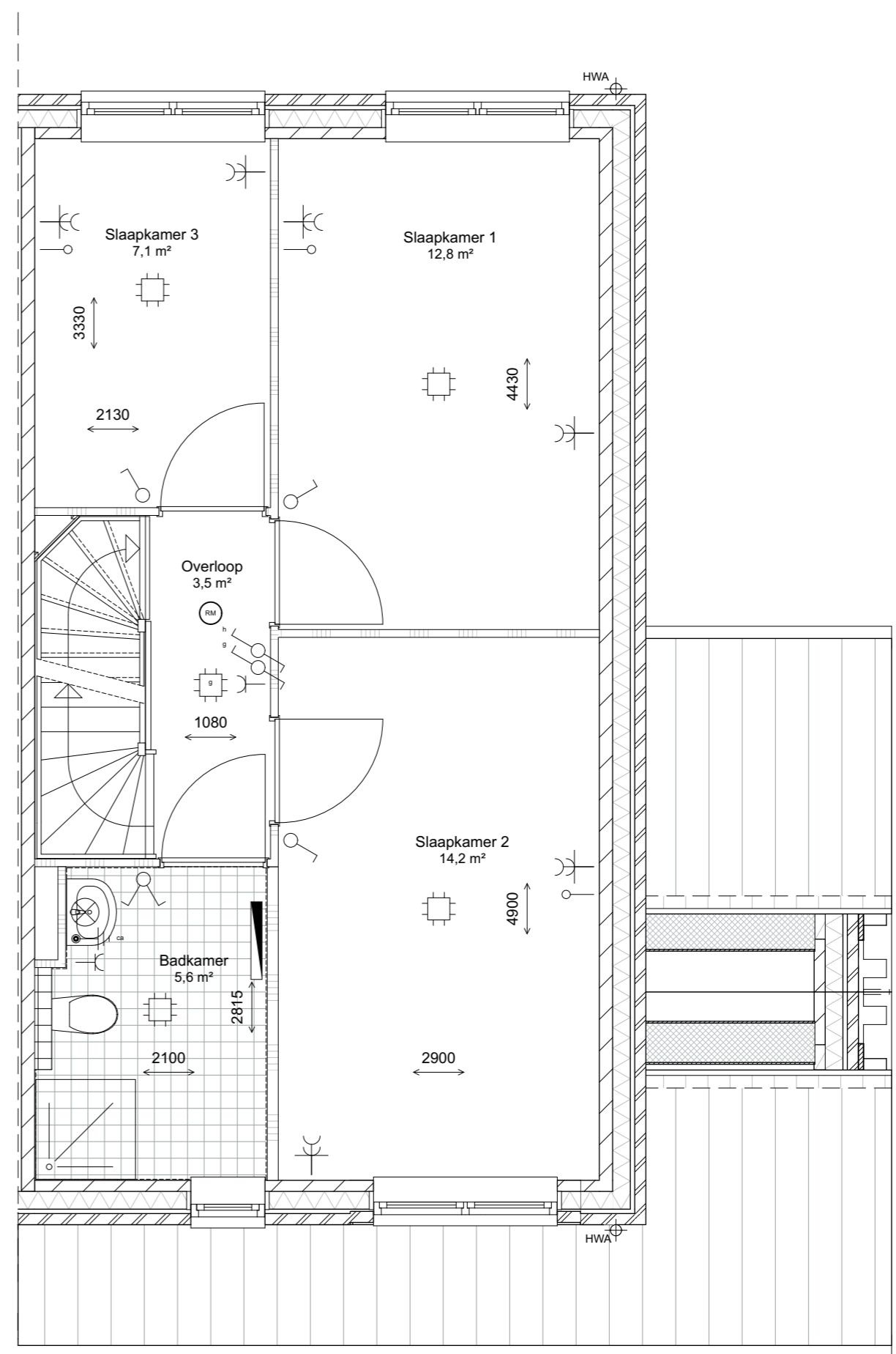
eerste verdieping 1:50
