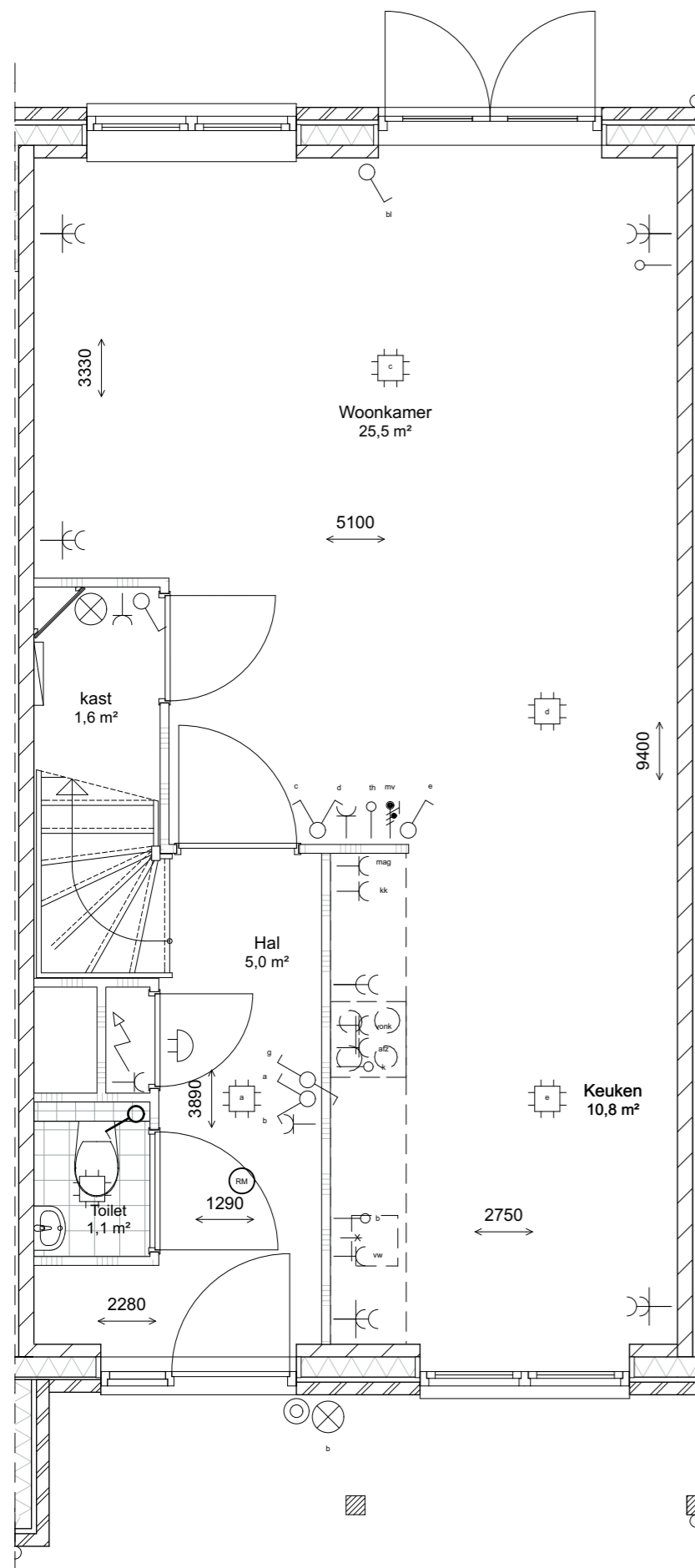
begane grond 1:50
