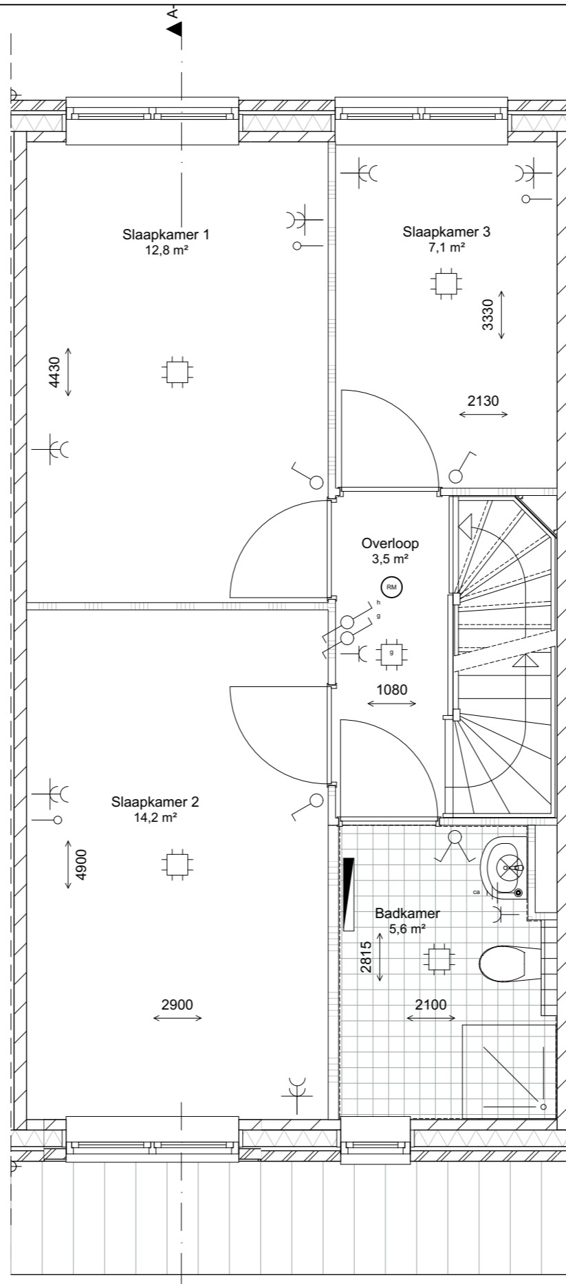
eerste verdieping 1:50
