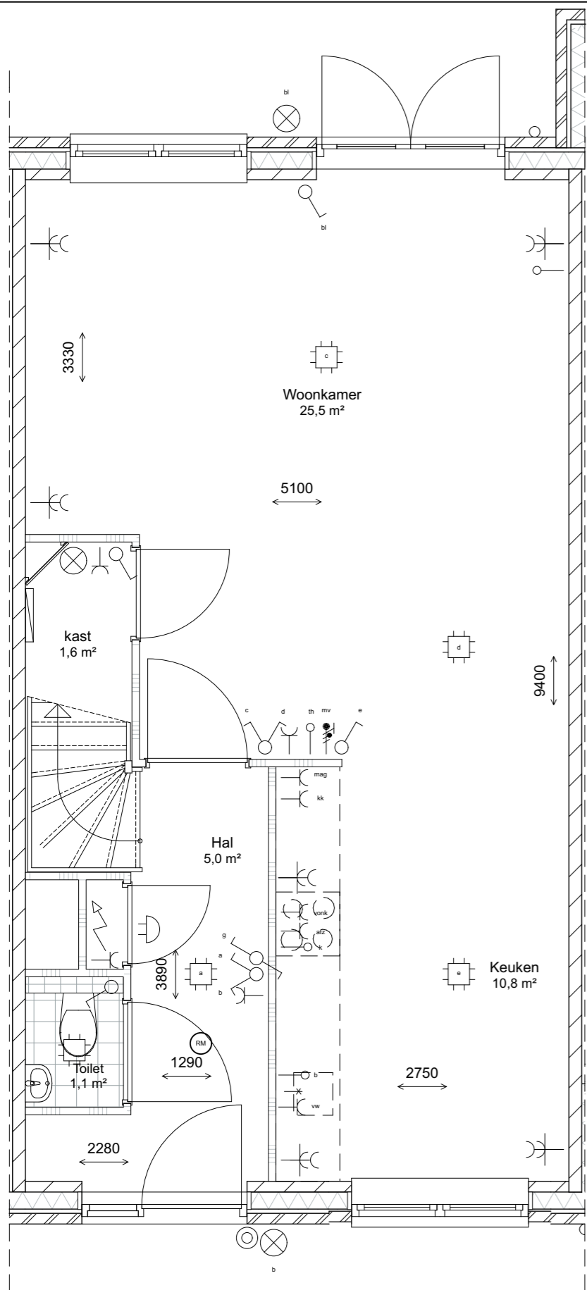
begane grond 1:50
