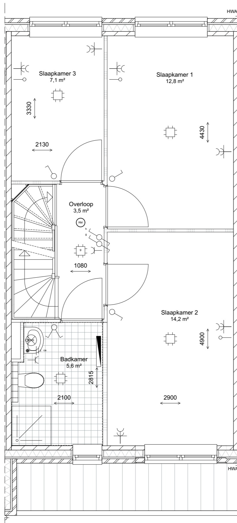
eerste verdieping 1:50
