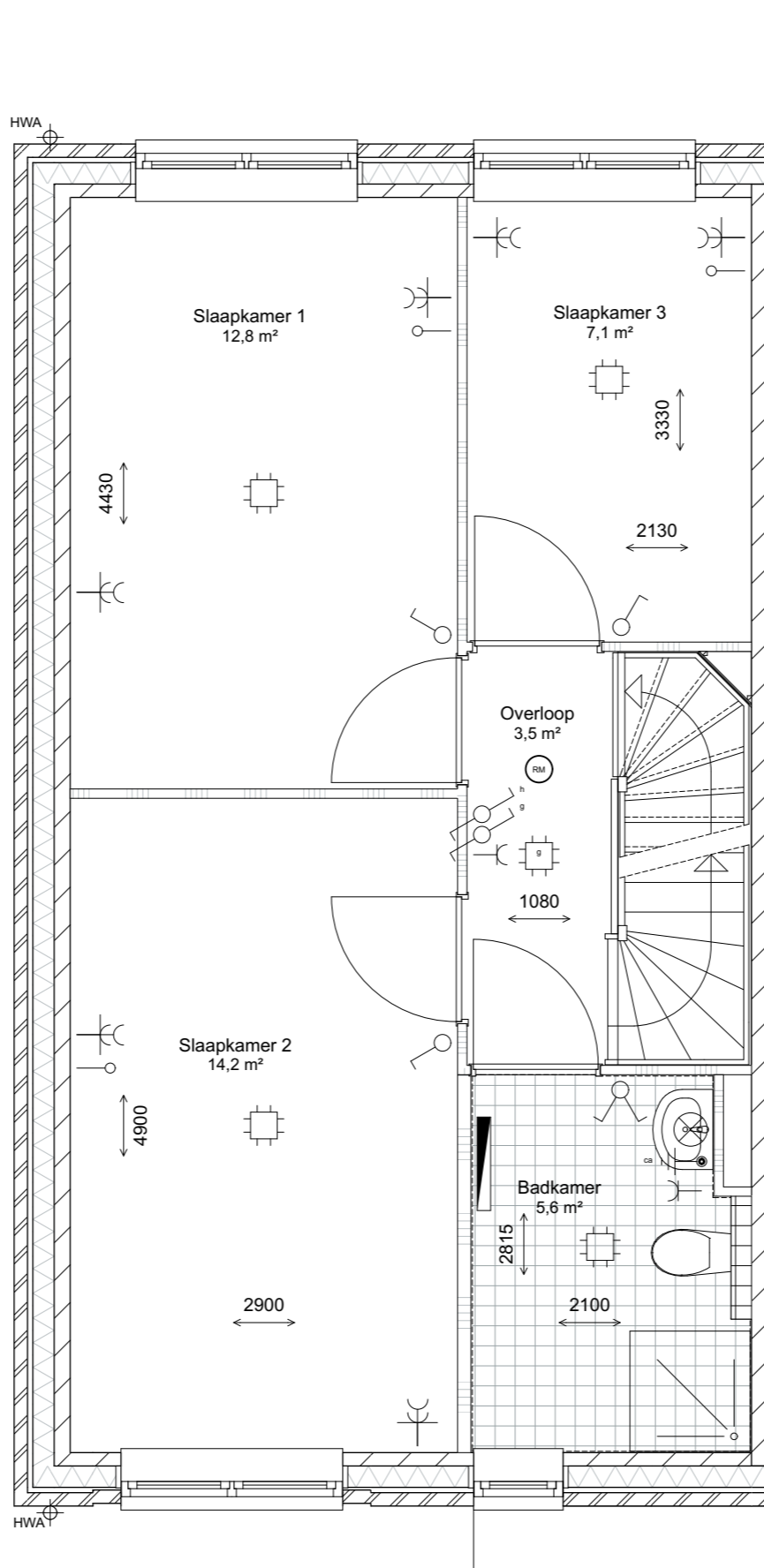
eerste verdieping 1:50
