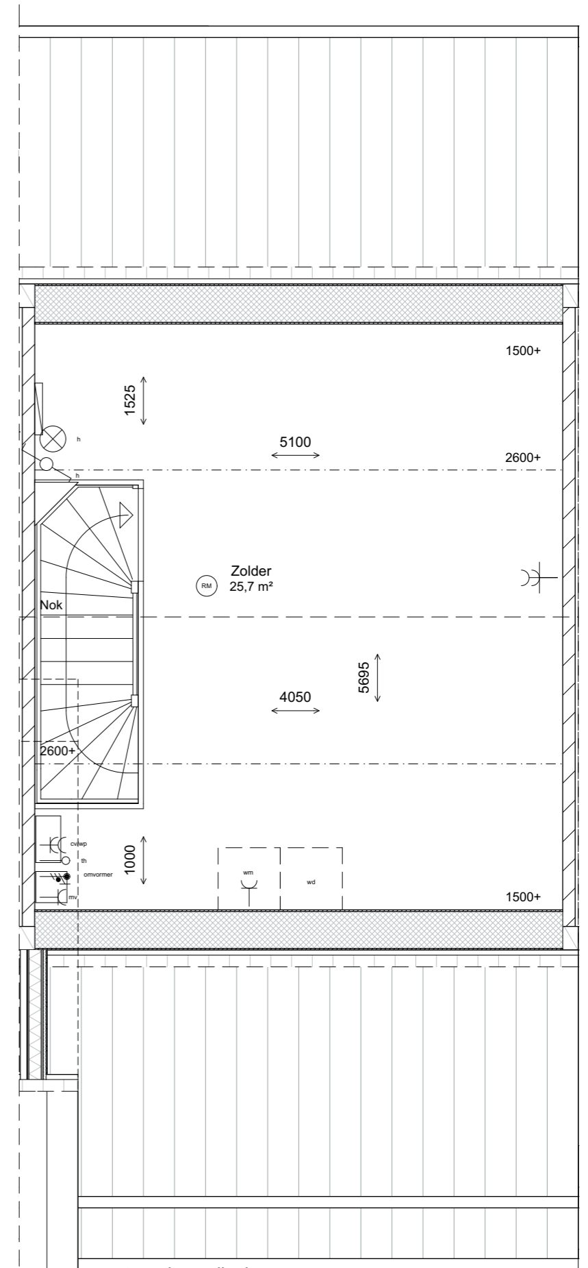
tweede verdieping 1:50
