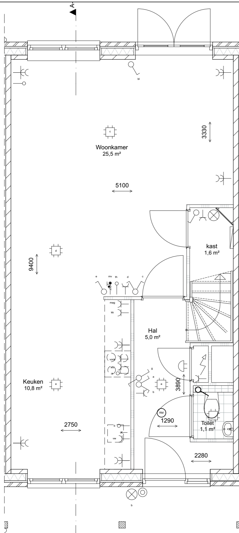
begane grond 1:50
