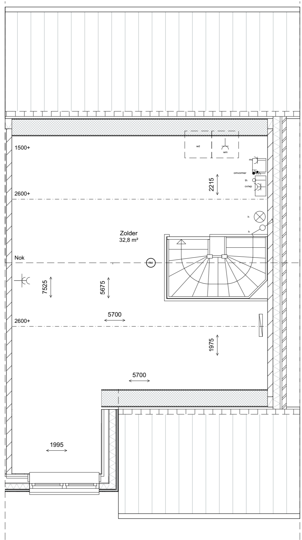
tweede verdieping 1:50
