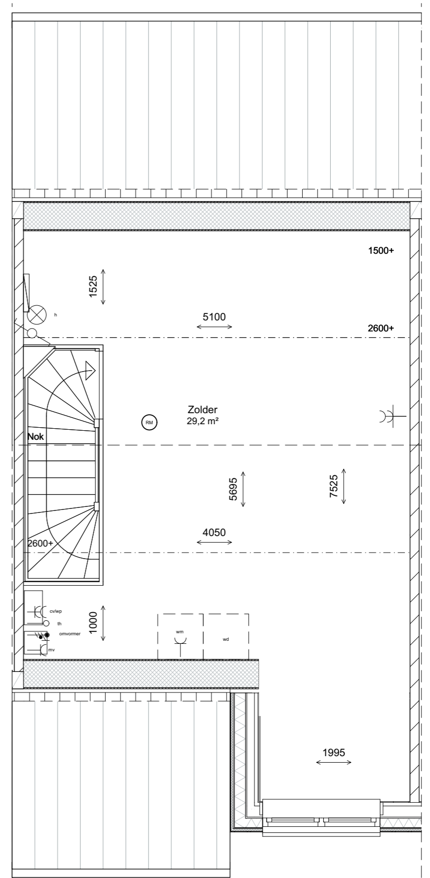
tweede verdieping 1:50
